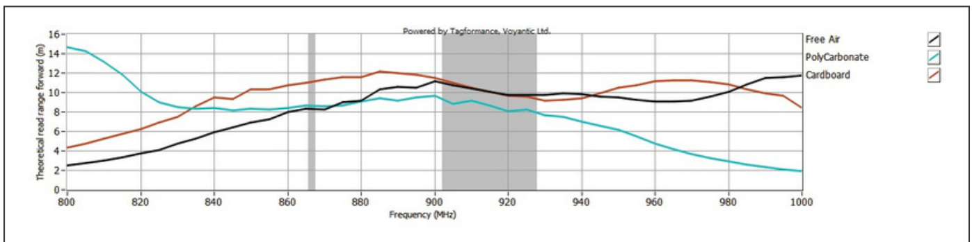
PID 4519 - RF performance(M730)
